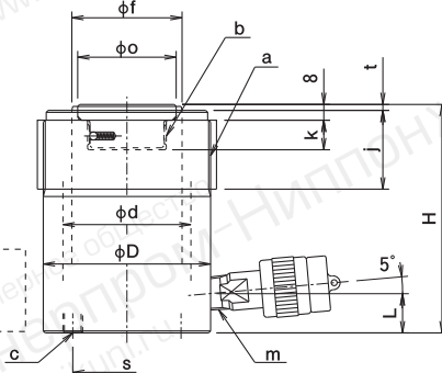
Габаритный чертёж
