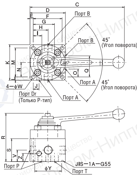
Габаритный чертеж
