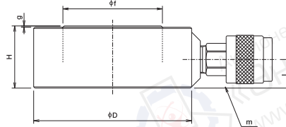
Габаритный чертеж
