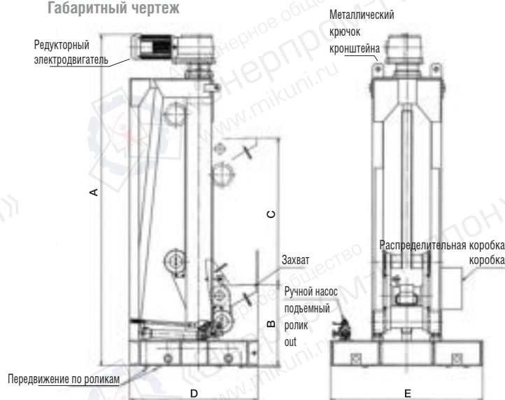
Габаритный чертеж
