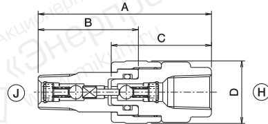
Габаритный чертеж
