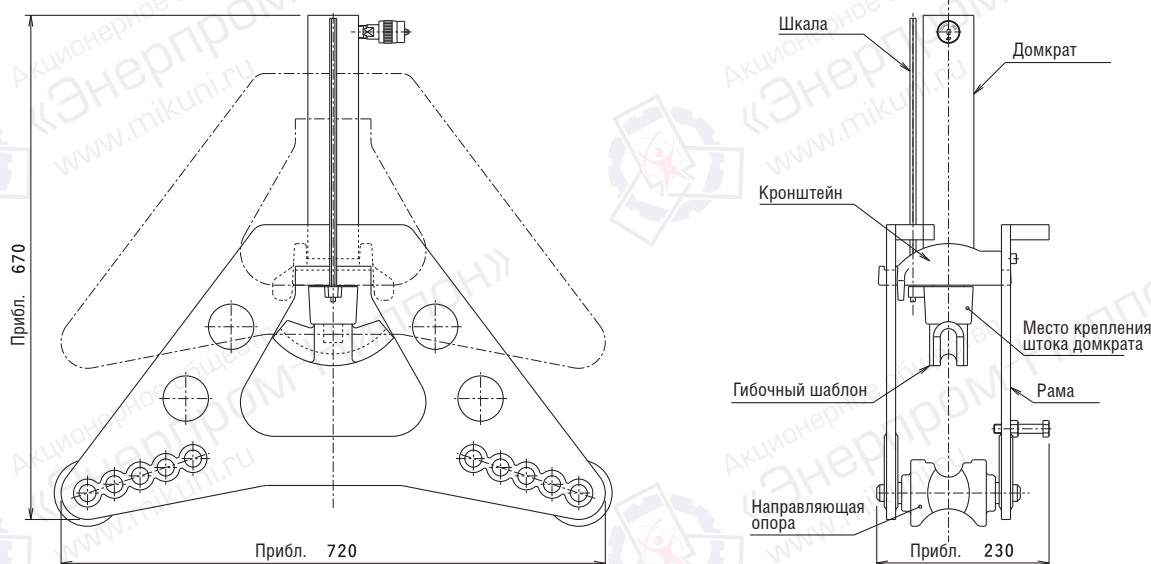
Габаритный чертеж
