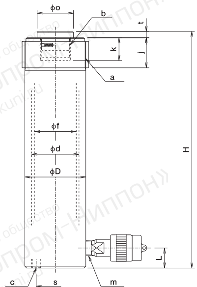
Габаритный чертеж
