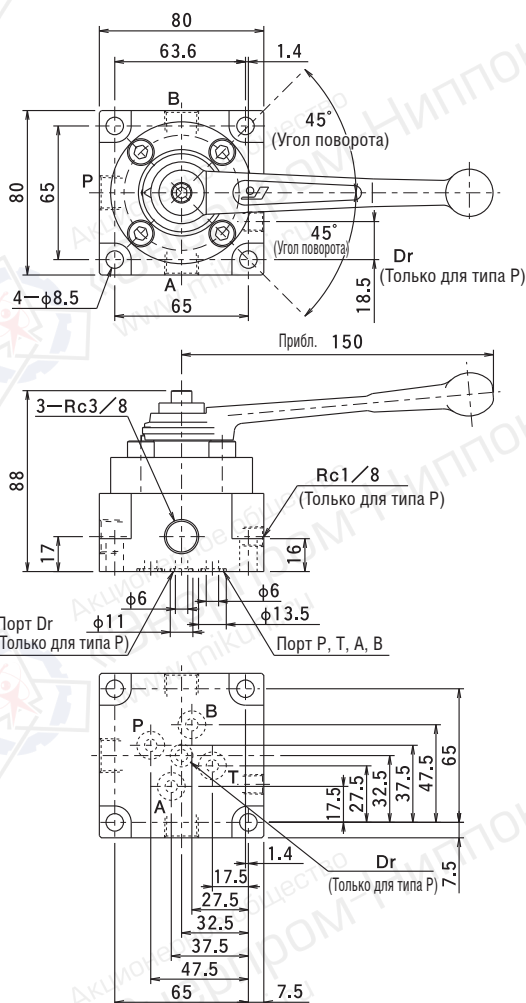
Габаритный чертеж
