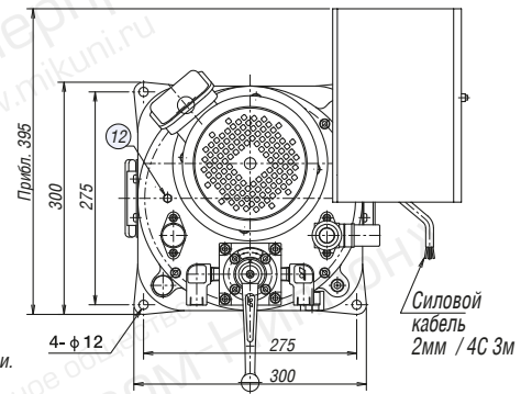
Габаритный чертеж с понижающим трансформатором
