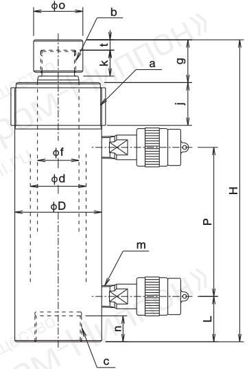
Габаритный чертеж
