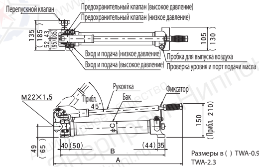
Габаритный чертеж
