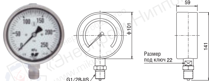
Габаритный чертёж
