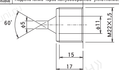
Резьбовое соединение фитинга BZ-4 с домкратом и РВД через конусообразное уплотнение.
