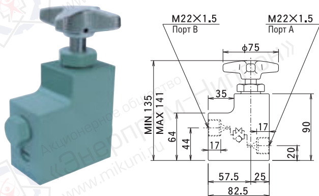
Габаритный чертёж
