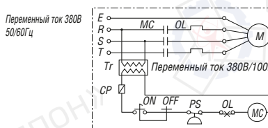
Электрическая схема с понижающим трансформатором
