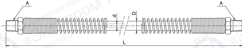
Резиновый рукав высокого давления RH
