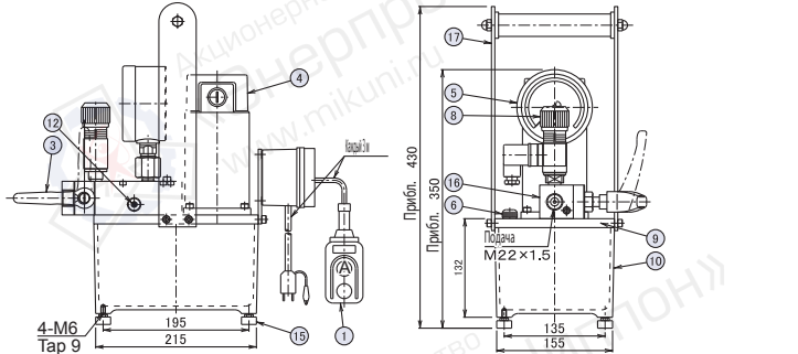
Габаритный чертеж
