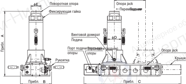
Габаритный чертеж
