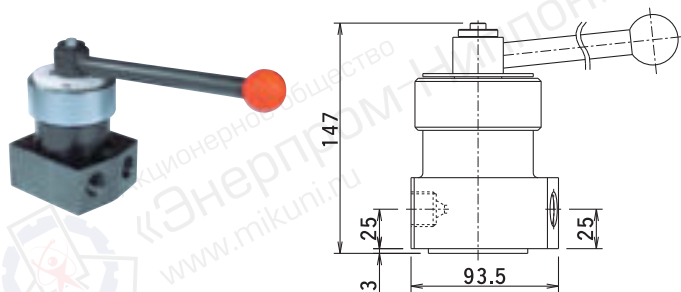
Габаритный чертёж
