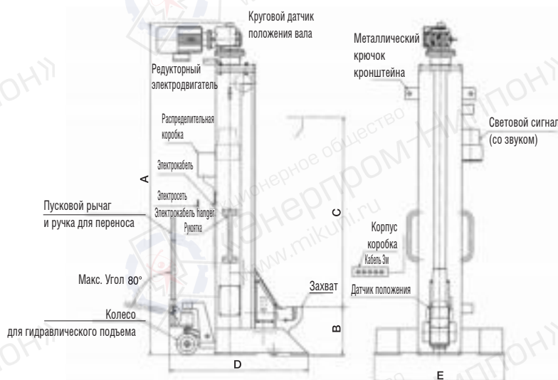
Габаритный чертеж
