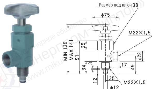
Габаритный чертёж
