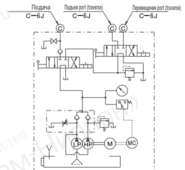
Схема гидросистемы
