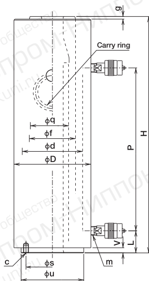
Габаритный чертеж
